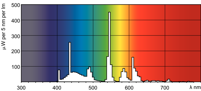
Designación de color /865
