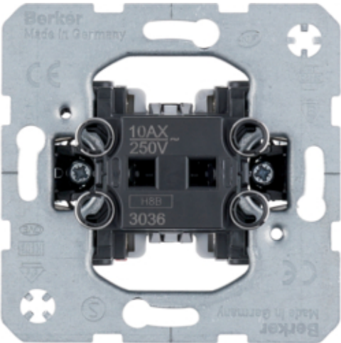
Conmutador 10AX, 250V
